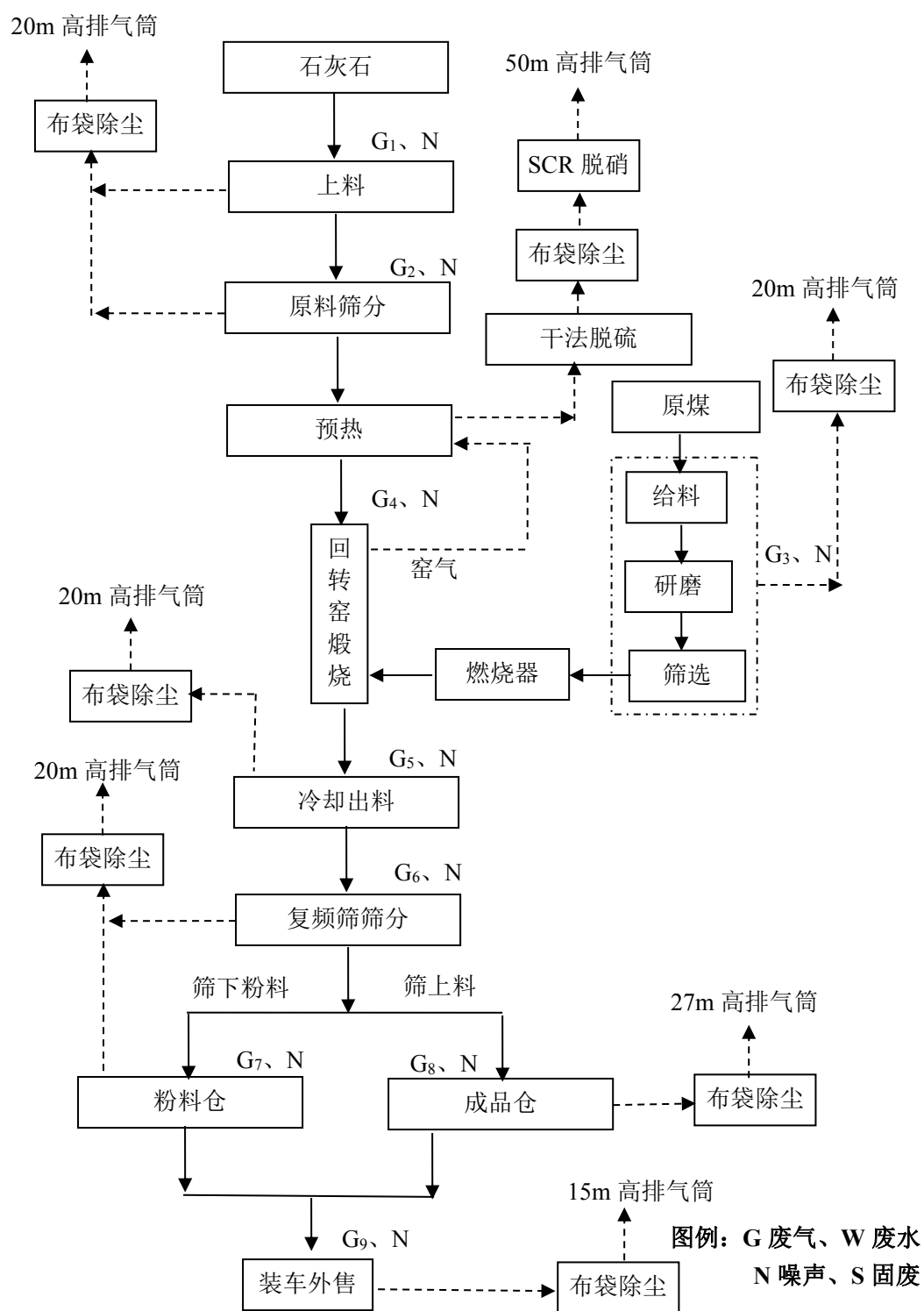
图 2-3 项目石灰生产流程及排污节点图
