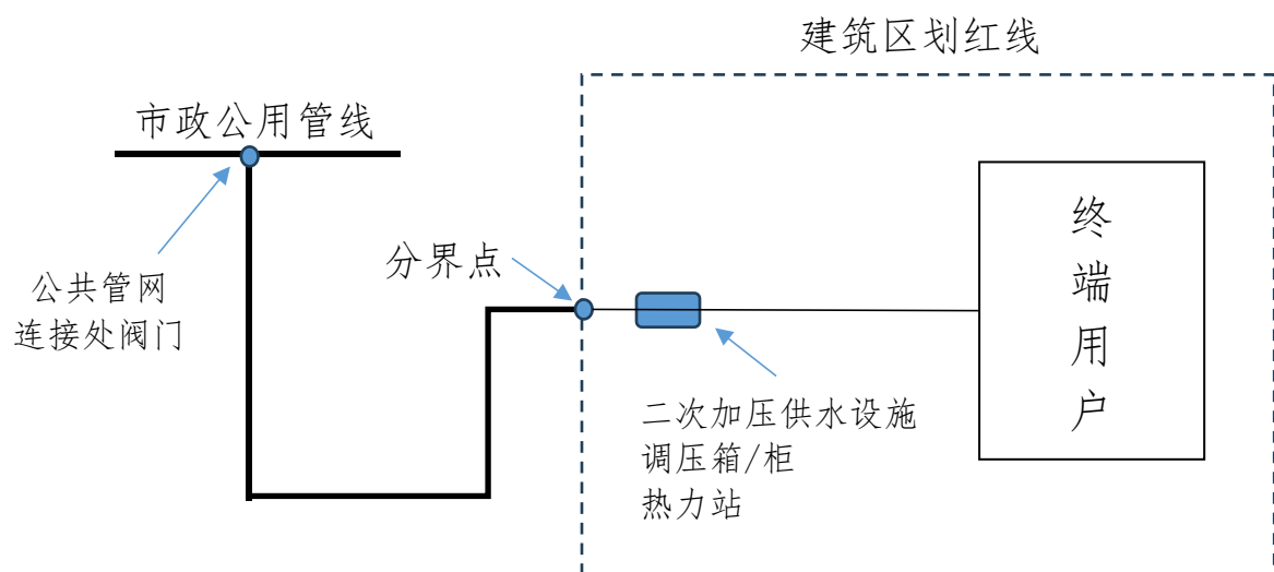
图 4 供水供气供暖接入工程范围
