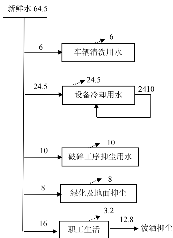
图 2-2 技改完成后全厂给排水平衡图 单位：m 3 /d
